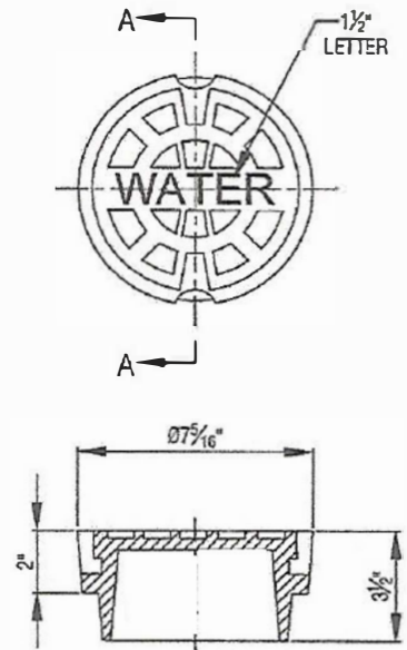
SECTION A-A LID
